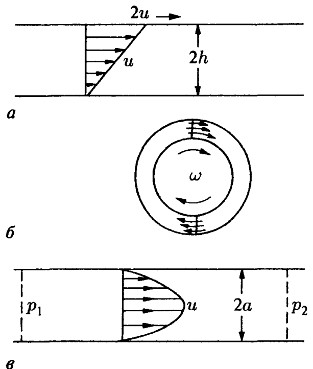
Рис. 4.6. Примеры конвективных систем, обнаруживающих неустойчивость при закритических вынуждающих силах: (а) плоское течение Куэтта; (б) течение Тейлора; (в) течение Пуазейля
