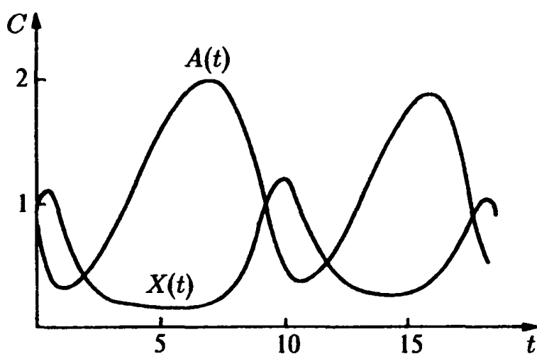
Рис. 4.26. Возникновение химических колебаний
