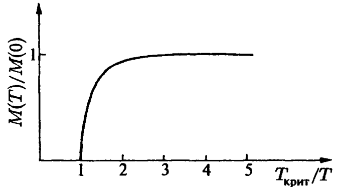
Рис. 5.6. Намагничивание ферромагнетика как функция температуры T ( T_{\text{крит}} — критическая температура)
