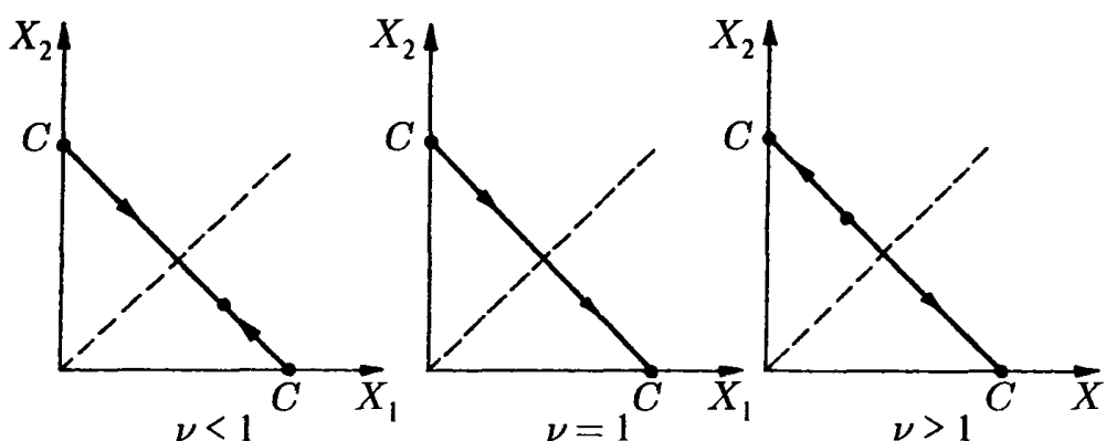
Рис. 5.23. Стабилизация при гиперболическом росте концентраций двух компонент и постоянной суммарной концентрации
