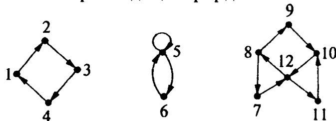
Рис. 6.9. Полностью разложимая каталитическая система
