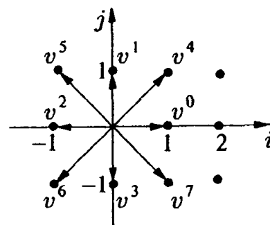
Рис. 5.12. Векторы разностей для обозначения соседей
