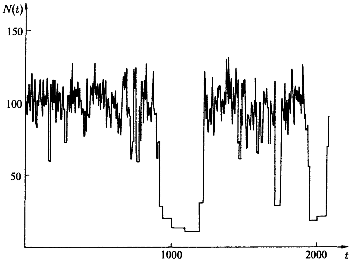
Рис. 5.34. Стохастическая траектория в модели Шлёгля
