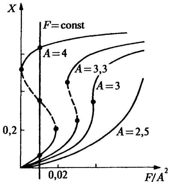
Рис. 4.25. «Провисание» графика зависимости стационарной концентрации X от F в бистабильной области
