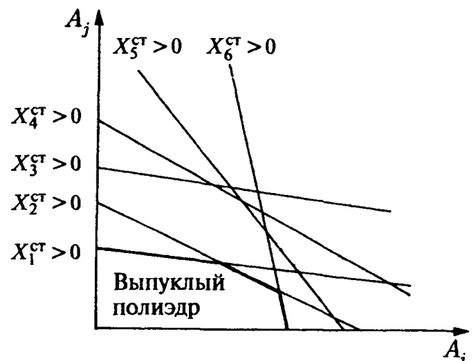
Рис. 6.20. Устойчивые состояния могут располагаться на поверхности выпуклого полиэдра
