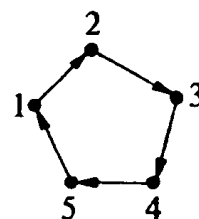
Рис. 6.8. Простой каталитический цикл
