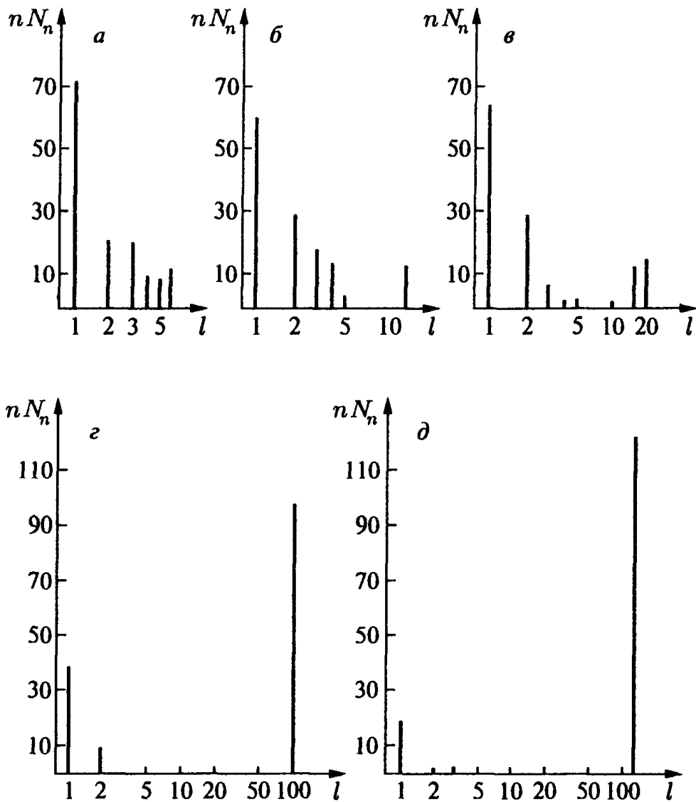
Рис. 4.2. Результаты моделирования (из работы: Schweitzer et al., 1988) образования кластеров в сильно пересыщенном паре ( t = 0, p/p' = 12,5 ): (а) t = 0,36, p/p' = 8,35 ; (б) t = 0,79, p/p' = 8,15 ; (в) t = 1,47, p/p' = 7,30 ; (г) t = 6,75, p/p' = 3,17 ; (д) t = 27,25, p/p' = 2,17
