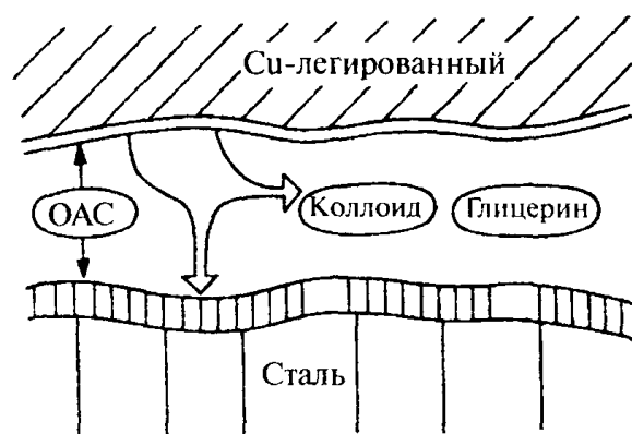
Рис. 12.4. Схема селективного трения по Гаркунову и Крагельскому при образовании диссипативных структур в слое трения
