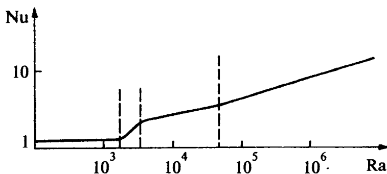
Рис. 4.13. Многократные изломы в зависимости числа Нуссельта от числа Рэлея при закритических значениях последнего при качественных изменениях механизма переноса тепла
