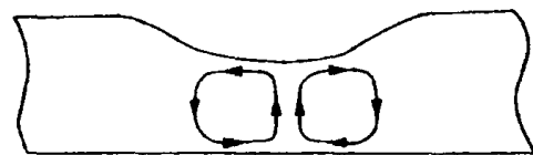
Рис. 12.3. Образование утоньшений в сохнущем лаковом покрытии на основе эффекта Марангони
