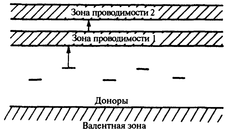
Рис. 4.18. Эффект Ганна: схема структуры полос в полупроводнике
