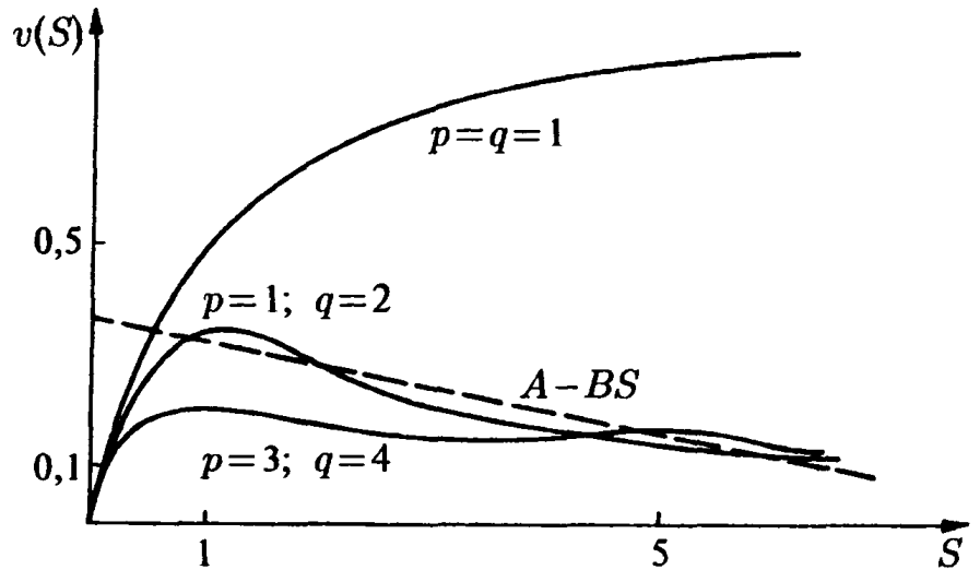
Рис. 5.26. Различные зависимости скорости ферментативной реакции v от концентрации субстрата S
