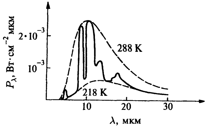
Рис. 3.5. Схема спектрального распределения земного излучения (Сватков, 1974)
