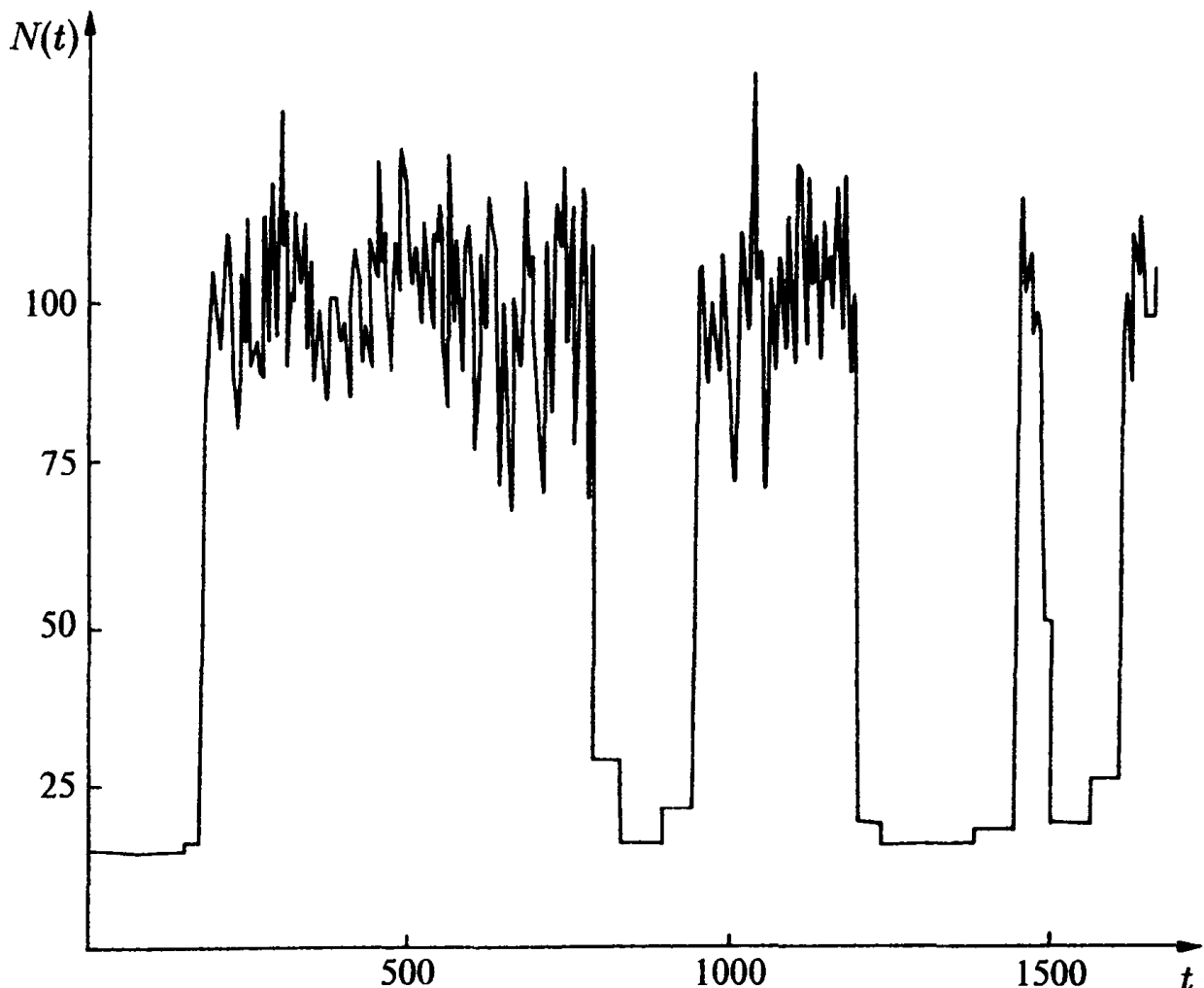
Рис. 5.33. Стохастическая траектория в модели Шлѐгля
