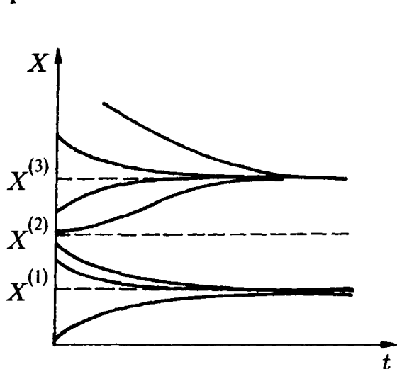
Рис. 5.21. Временная зависимость решений в бистабильной модели Шлёгля
