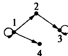
Рис. 6.12. Каталитический каскад (элементарный разложимый)
