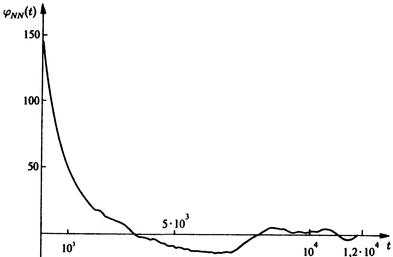
Рис. 5.37. Автокорреляция в стохастической модели Шлёгеля
