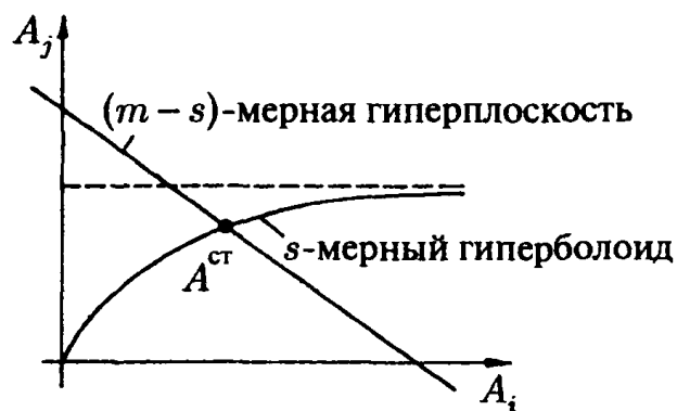
Рис. 6.19. Стационарное состояние сосуществования s сортов в пространстве сырья
