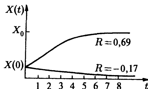
Рис. 5.4. Логистический рост (закон Ферхюльста—Перла)
